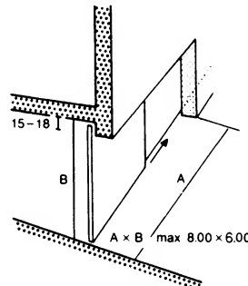
7 Sliding door (steel T30-T90)
